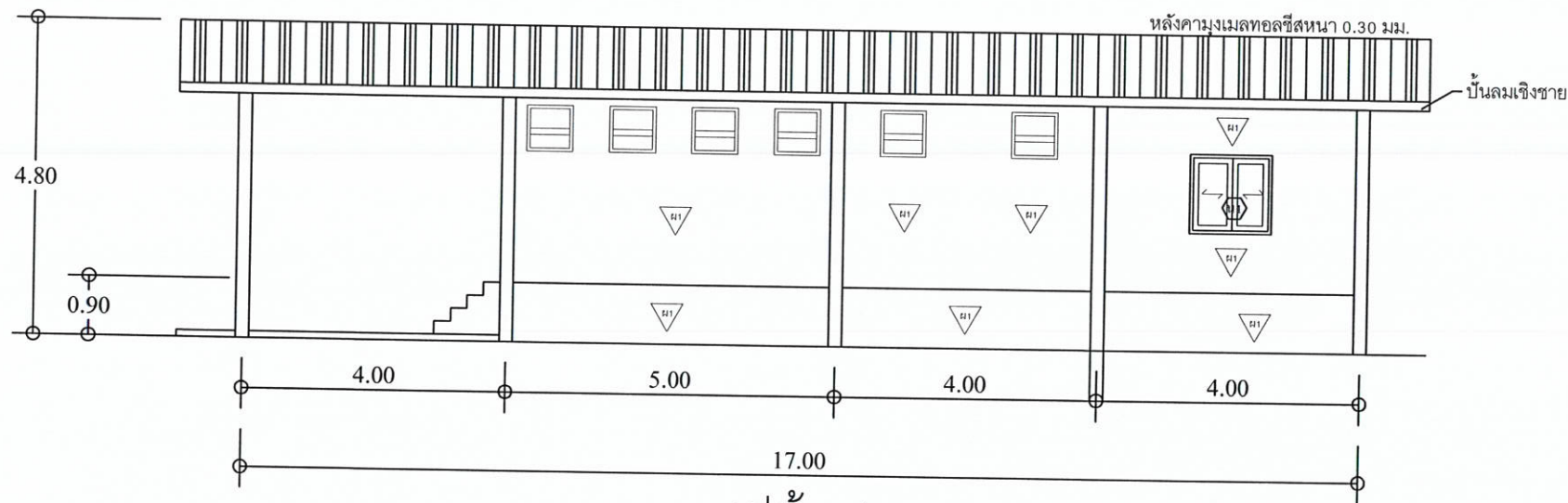
รูปด้าน 4 Scale 1:100
