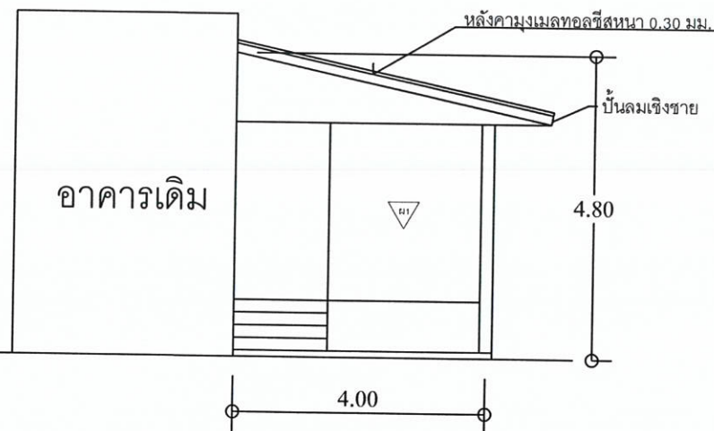
รูปด้าน 3 Scale 1:100
