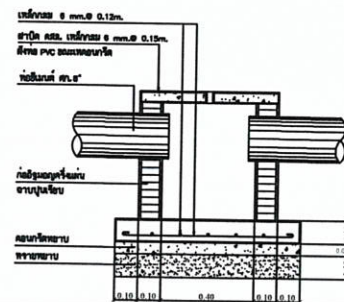
รูปตัดป่อพักน้ำทิ้ง No Scale
