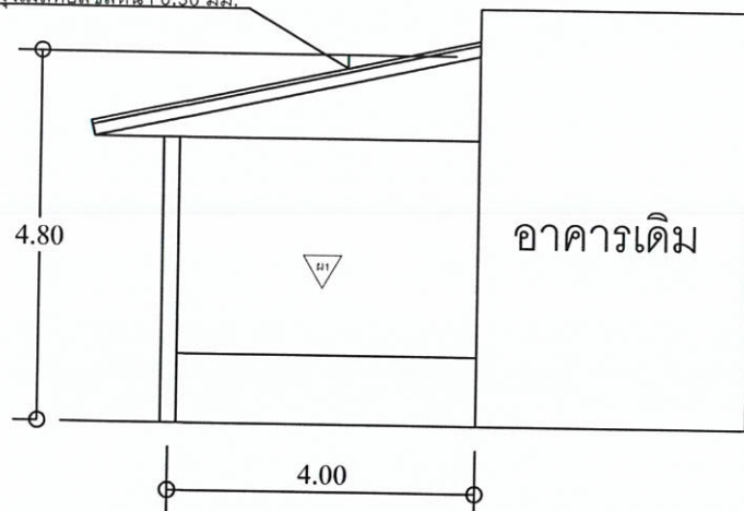
รูปด้าน 2 Scale 1:100
