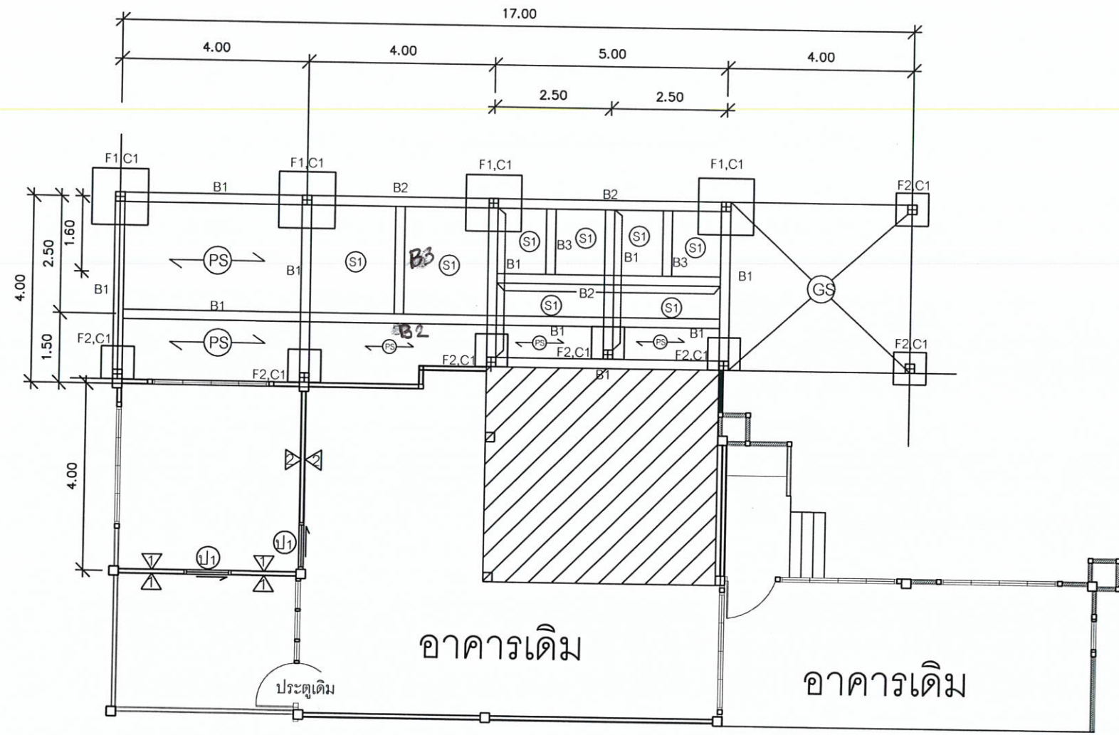
แปลนฐานราก,เสา,คาน พื้น ชั้น 1 มาตราส่วน 1 : 100
