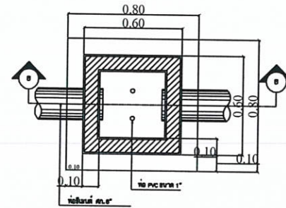
มั่งป่อพักน้ำทิ้ง No Scale
