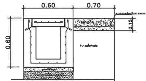
ภาพตัดแสดงรายละเอียด ฝิวทาง คสล.
