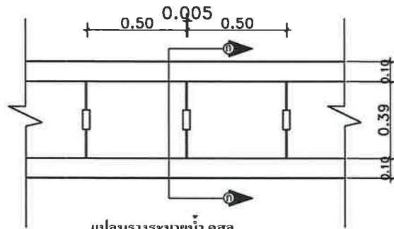
แปลนรกระจายน้ำ คสล.
