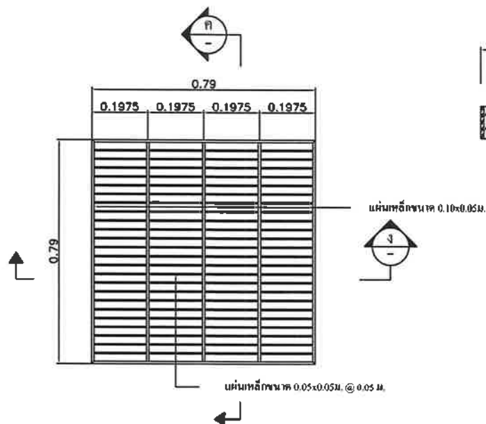
แปลนฝาปิดบอร์รับน้ำตะแกรงเหล็ก มาตราส่วน 1:10
