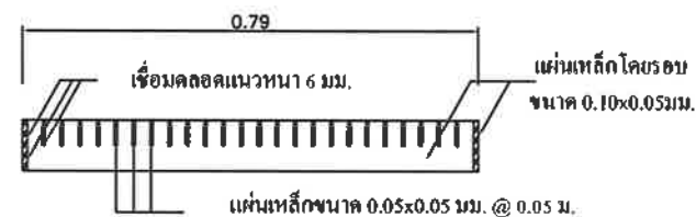
รูปตัด ก มาตราส่วน 1:10
