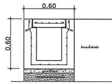
ภาพตัดแสดงรายละเอียด ผิวทาง คสล.
