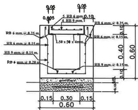
ภาพตัดแสดงรายละเอียดเหล็กเสริมราง คสล.
