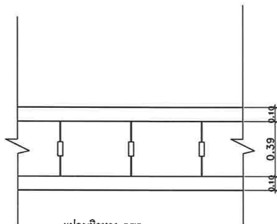
แปลนผิวทาง คสล.
