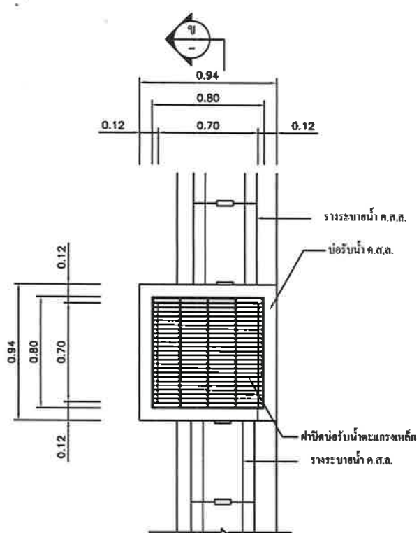
แปลนบอร์รับน้ำ ค.ส.ล. มาตราส่วน 1:20
