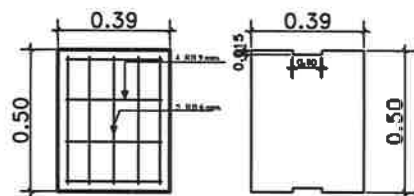
รายละเอียดเหล็กเสริมฝาราง คสล.
