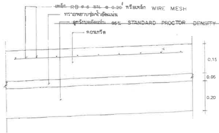
รายละเอียดคอนกรีตเสริมเหล็ก
