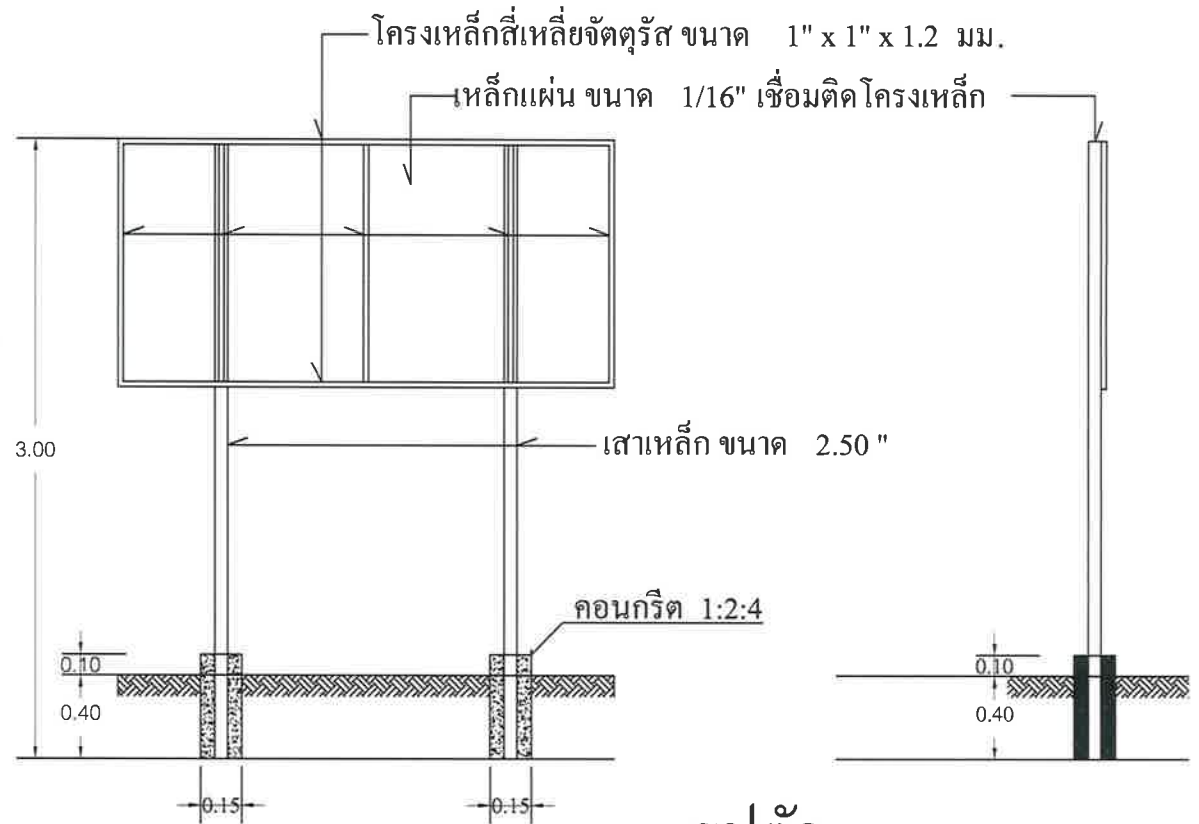
รูปตัด
