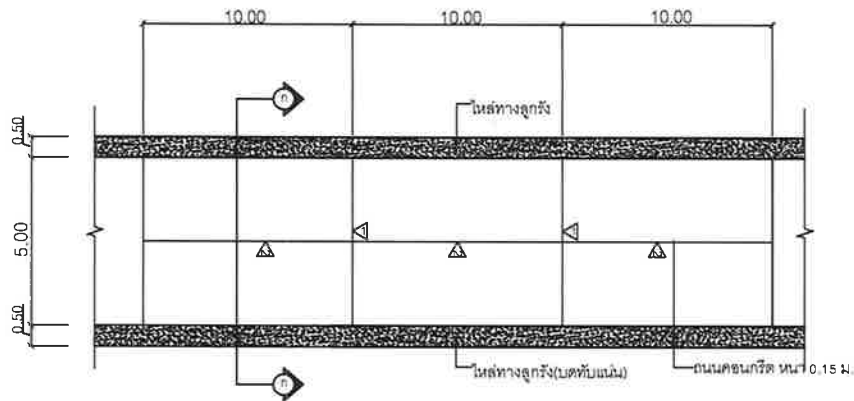
แบบรูปตัดมาตรฐาน ถนนคอนกรีต เสริมเหล็ก ขนาด 5.00 เมตร
