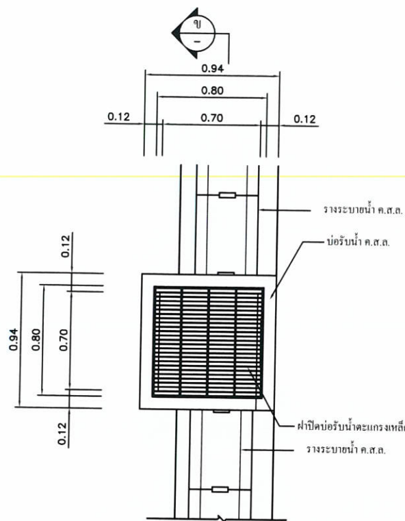
แปลนบ่อน้ำ ค.ส.ล. มาตราส่วน 1:20
