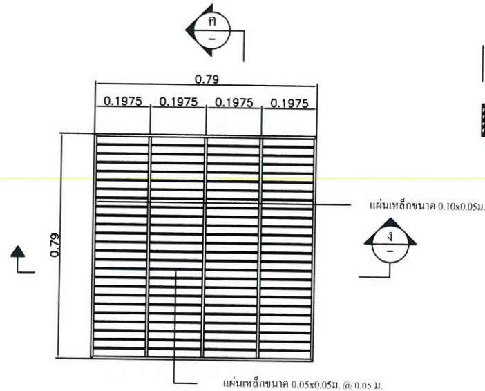
แปลนฝาปิดบ่อน้ำตะแกรงเหล็ก มาตราส่วน 1:10
