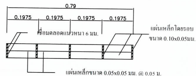
รูปตัด ง มาตราส่วน 1:10
