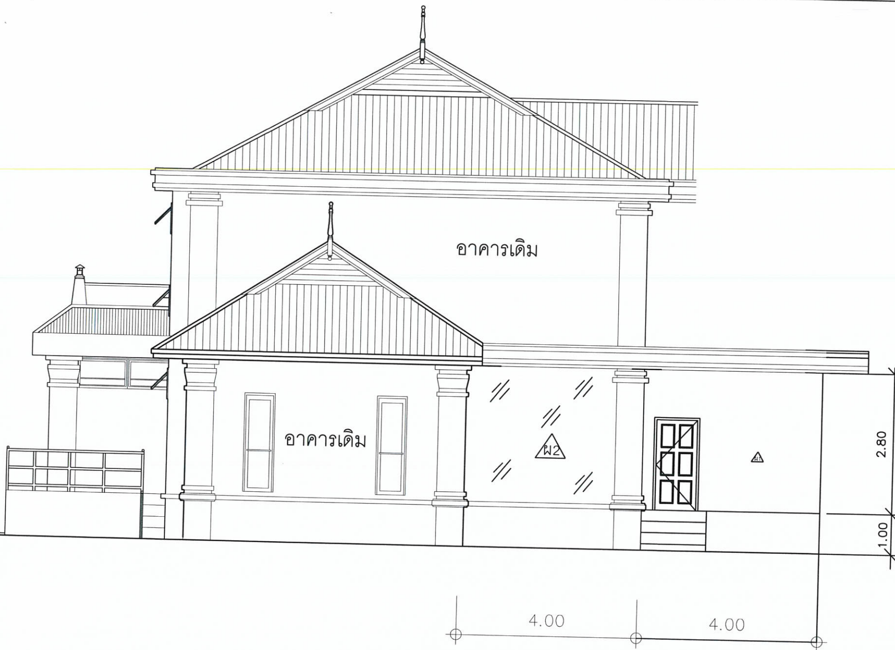
รูปด้าน 2 Scale 1:100
