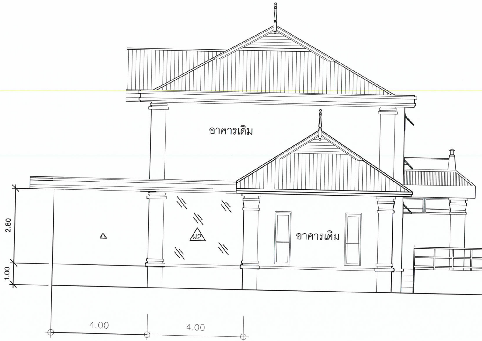
รูปด้าน 3 Scale 1:100
